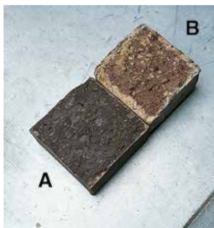
Obr. 2B: Skúšobný test - prienik chloridových iónov (UNI 9944). Vzorka A ošetrovaná Mapelasticom – bez priesaku; vzorka B neošetrovaná Mapelasticom - znázornenie pokročilého prieniku do niekoľkých mm
