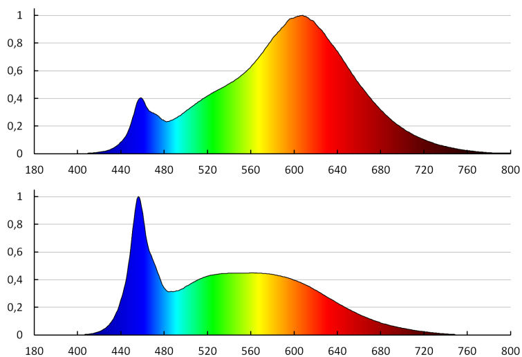
KANLUX S.A. (kat 33640) S A60 7W E27 CCT / LDC (Polar)
