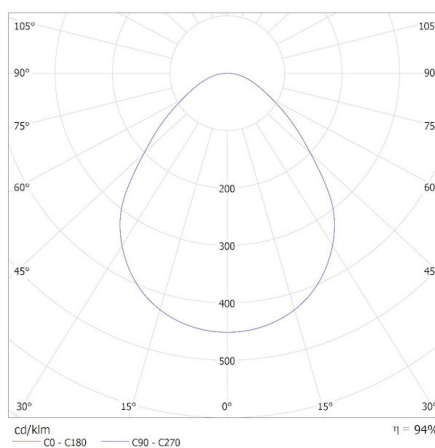
KANLUX S.A. (kat 26778) AVAR U 6060 32W-NW / Krzywa rozsyłu światła (biegunowo)
