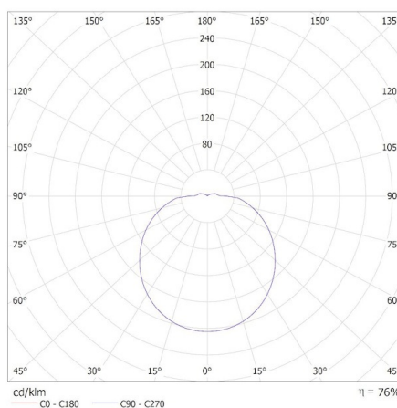
KANLUX S.A. (kat 26785) AVAR O 6060 40W-NW / Krzywa rozsyłu światła (biegunowo)
