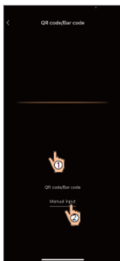
Obr.18 Skenovanie
