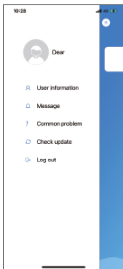
Obr.5 Ponuka vľavo
