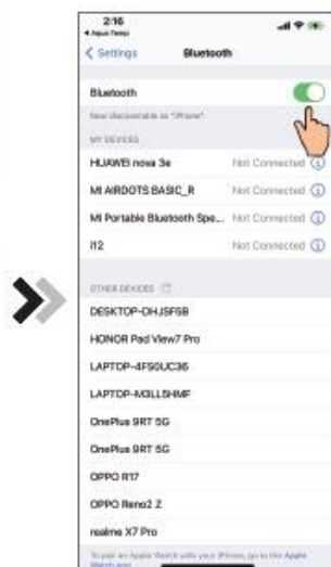
Obr.12 Bluetooth nastavenie
