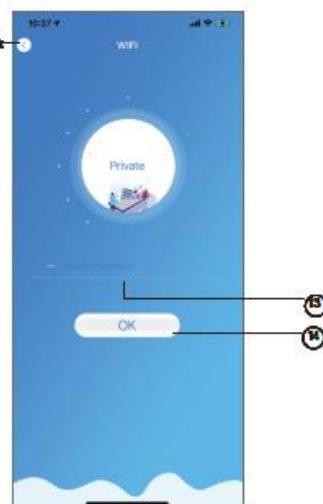
Obr.9 Vloženie hesla
