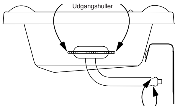
Åbninger i brænderens Venturi-rør
