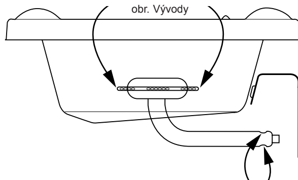
Otvory Venturiho trubky horáka
