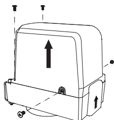
Obrázek 5 Odstranění krytu
