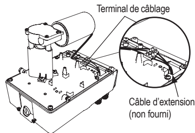
Image 7 Unité secondaire
