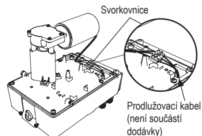
Obrázek 7 Sekundární jednotka
