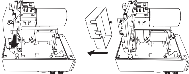
Abbildung 6 Primäreinheit
