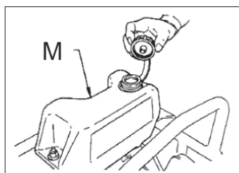
Kraftstofftank
