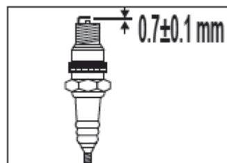
Provjera svjećice za
