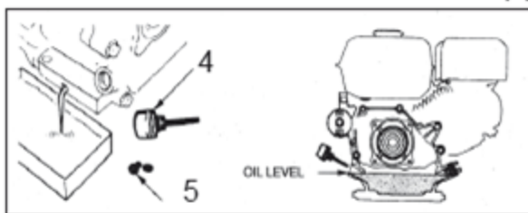
Promena motornog ulja
