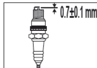
Zündkerze prüfen
