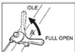
Ručica gasa/prazni hod „IDLE“
