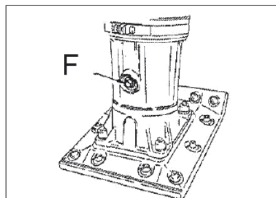
Schauglas / Ölablassschraube
