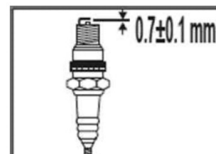
Provera svećice
