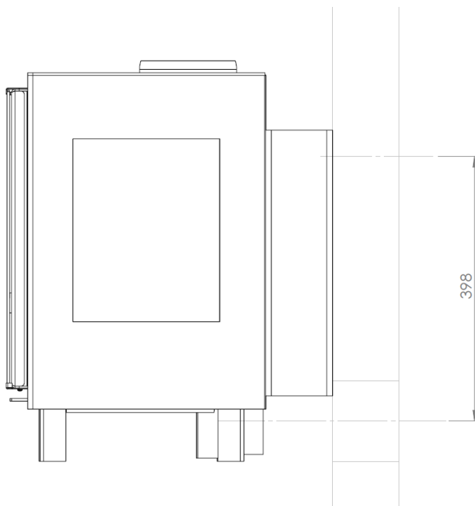
Ilustracja 4. Rysunek dołotu powietrza z zewnątrz
