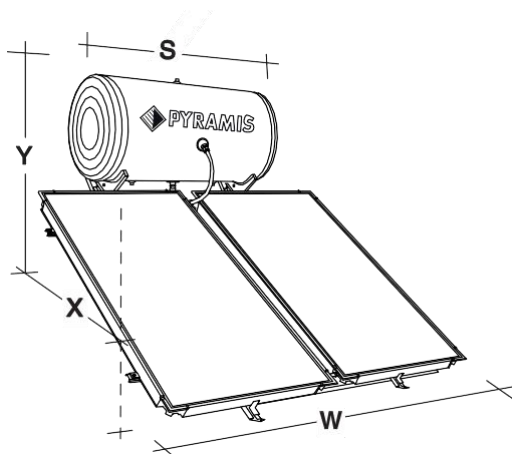
Rozmery kompletného solárneho systému v centimetroch (cm)
