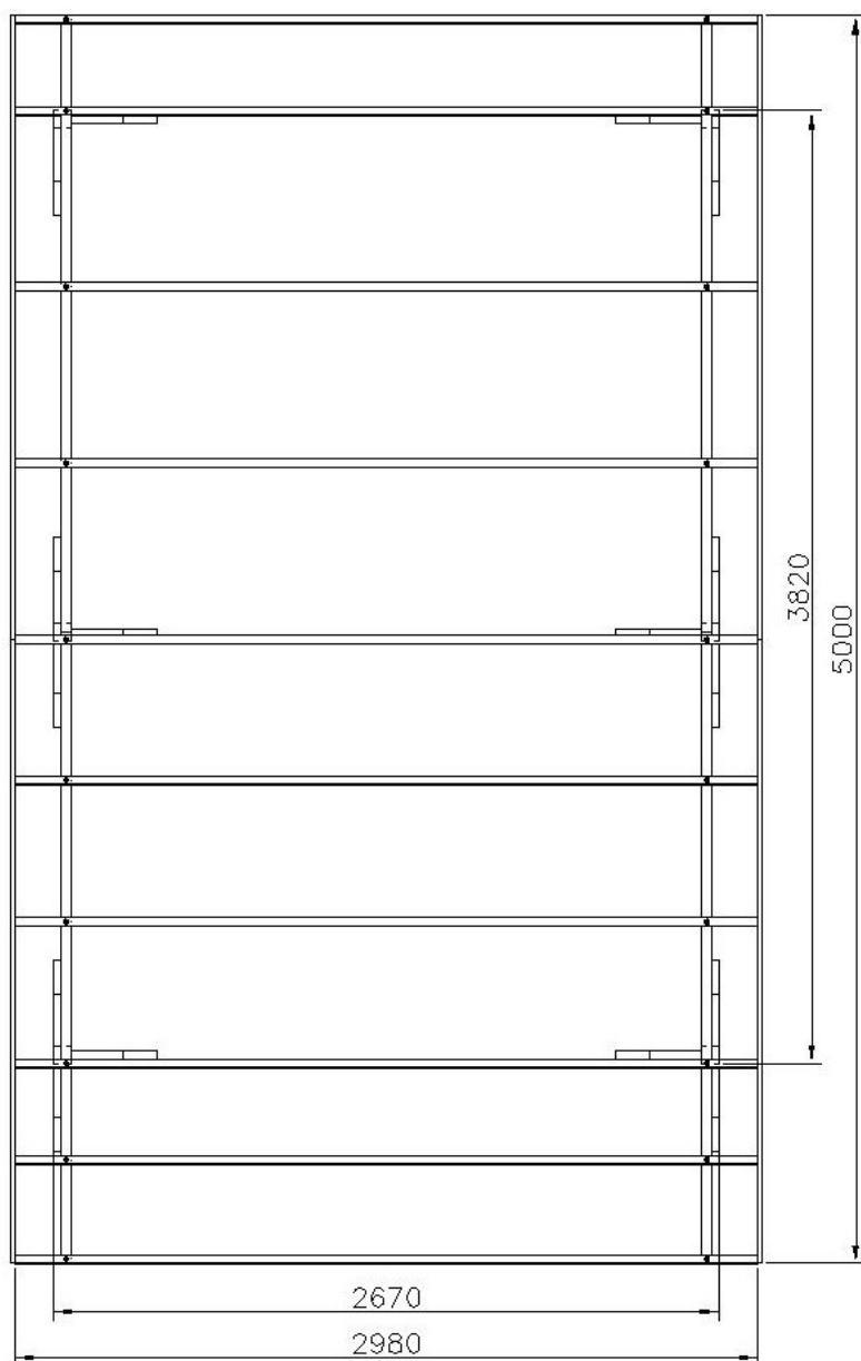
PŮDORYS
