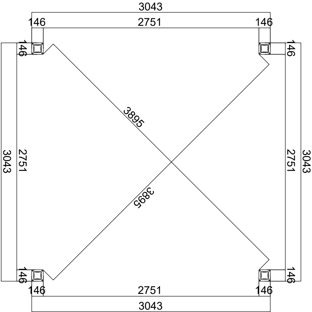
Schéma půdorysu základů - Base Plate Layout Plan
