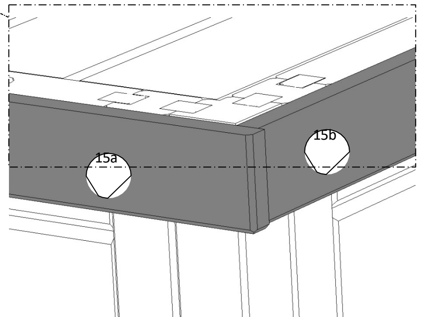
DETAIL V ROHU KRYCEJ LIŠŤY
