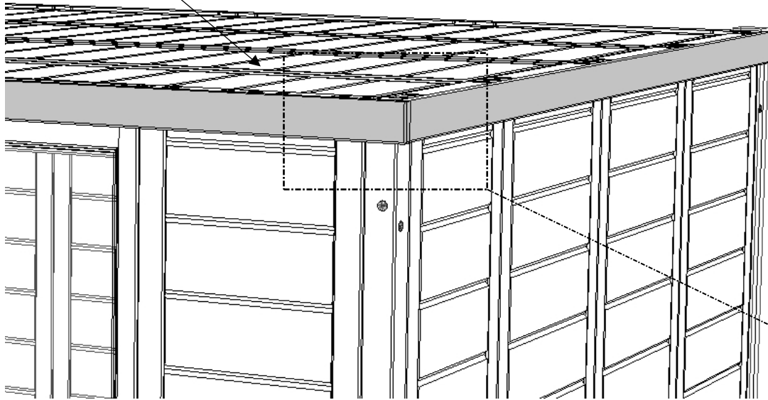
DETAIL REZU NA UPEVNIENIE KRYCÍCH LIŠŤ
