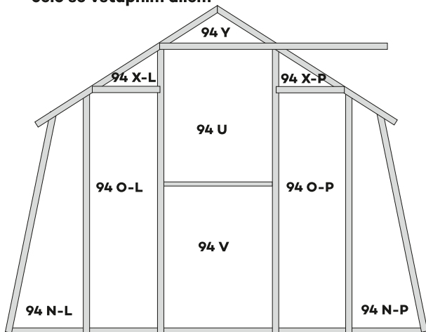
čelo se vstupním dílem
