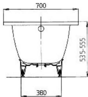
SANIFORM PLUS 362-1
