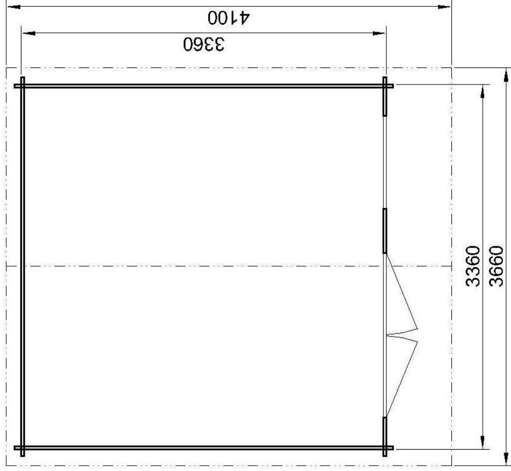
PÔDORYS
