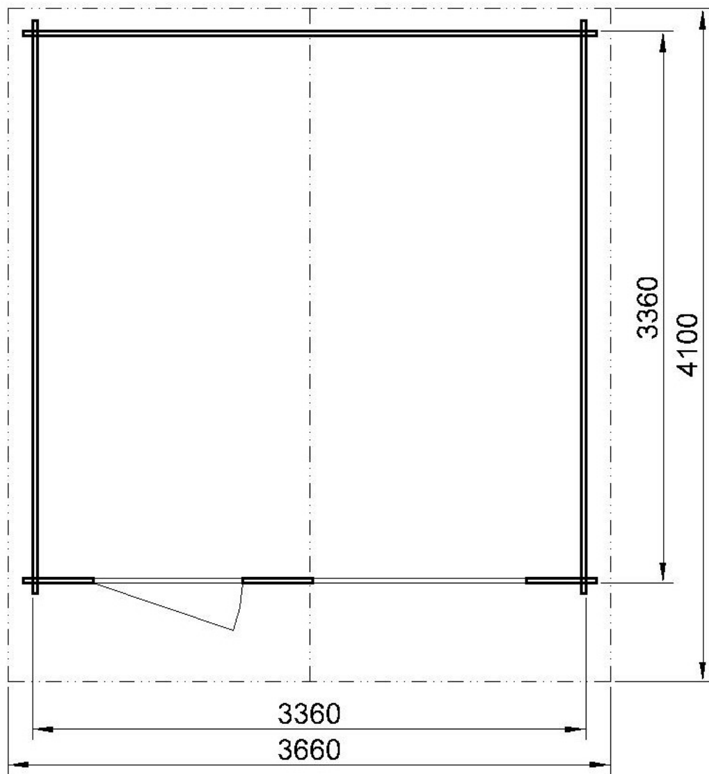
PÔDORYS
