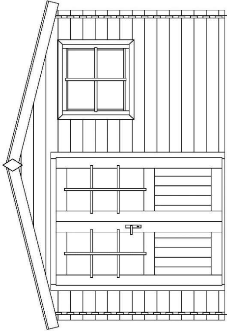
PREDNÝ POHĽAD
