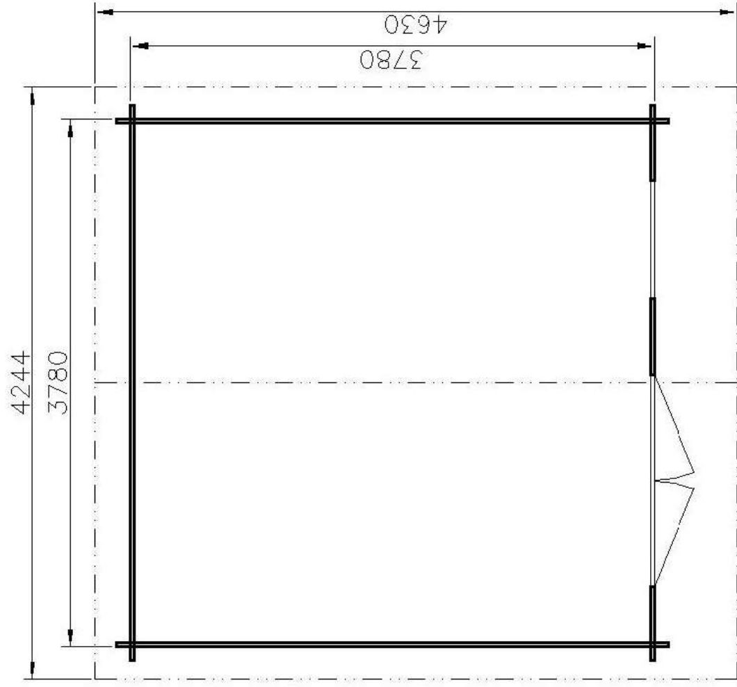
PÔDORYS
