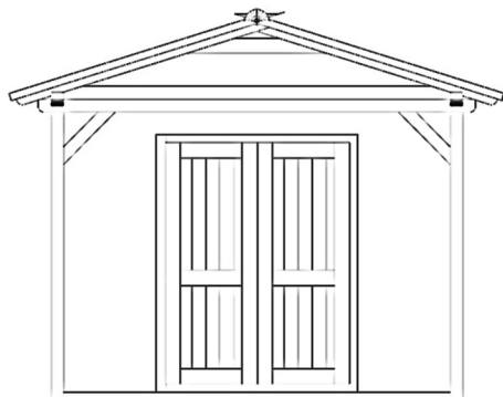
PREDNÝ POHĽAD
