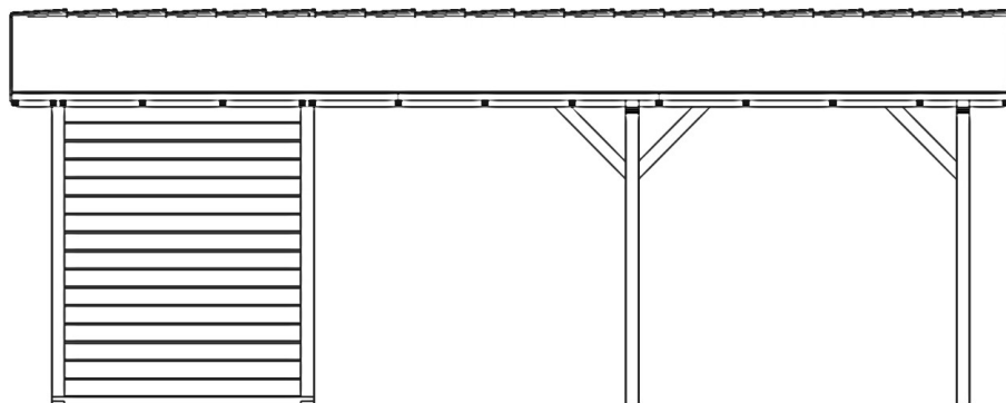
BOČNÝ POHĽAD ĽAVÝ
