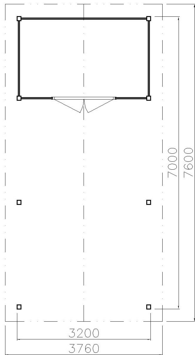
PODORYS
