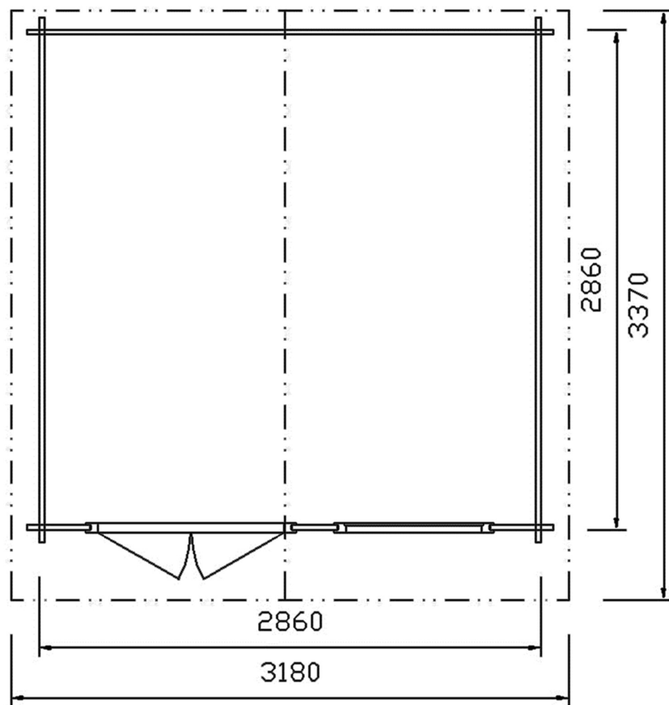
PÔDORYS
