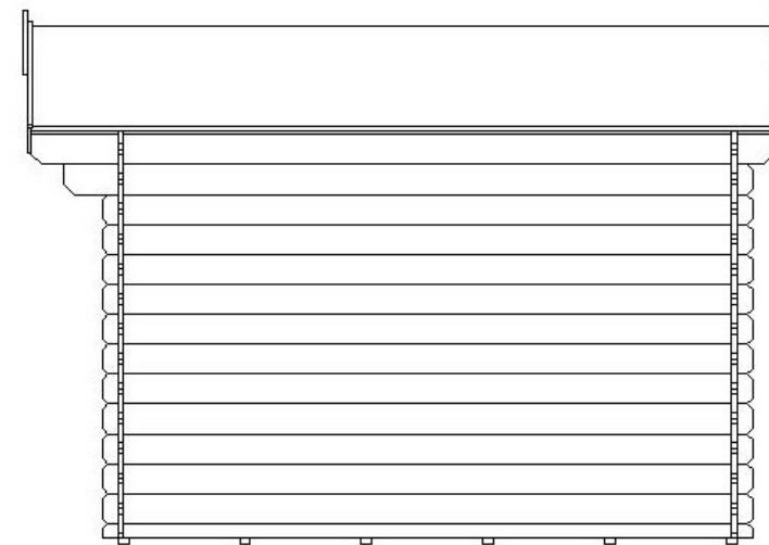
BOČNÝ POHĽAD PRAVÝ
