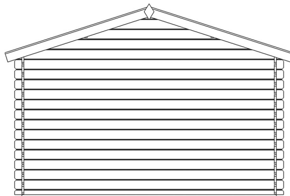
ZADNÝ POHĽAD
