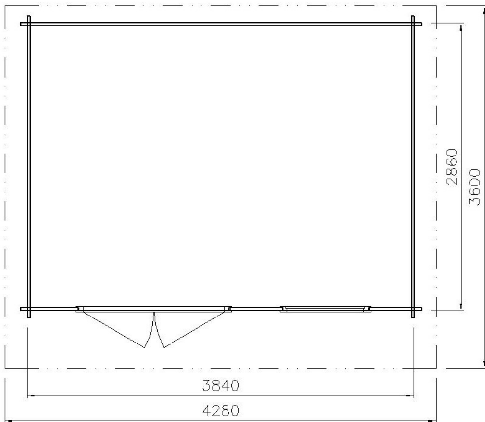
PÔDORYS
