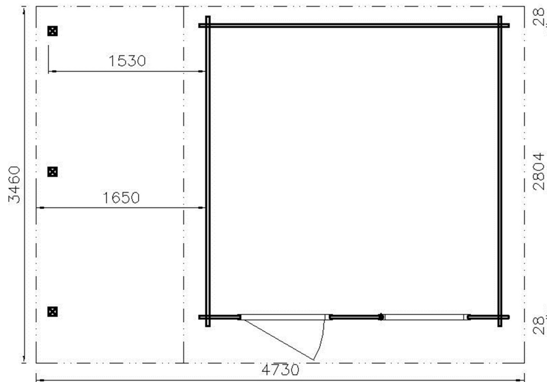
PÔDORYS
