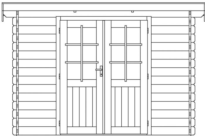
PREDNÝ POHĽAD
