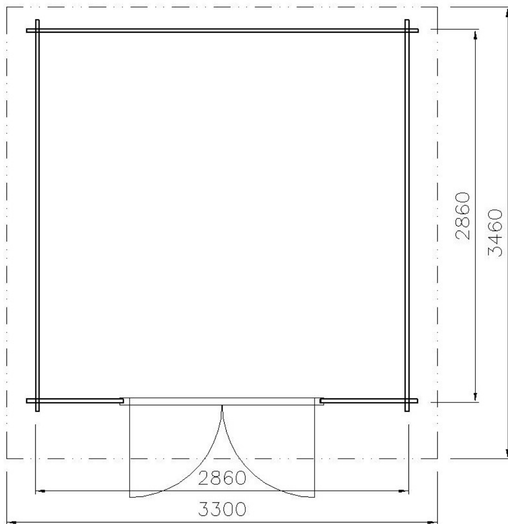
PÔDORYS
