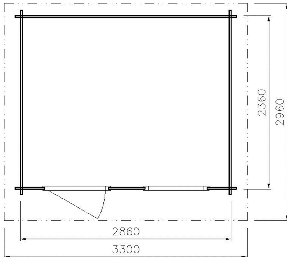
PÔDORYS
