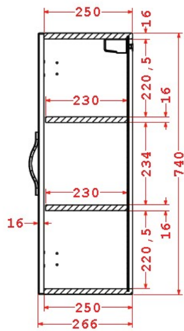
SEZIONE A-A
