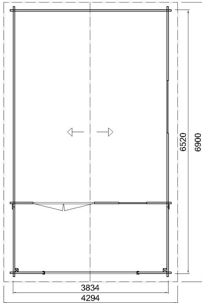
PÔDORYS
