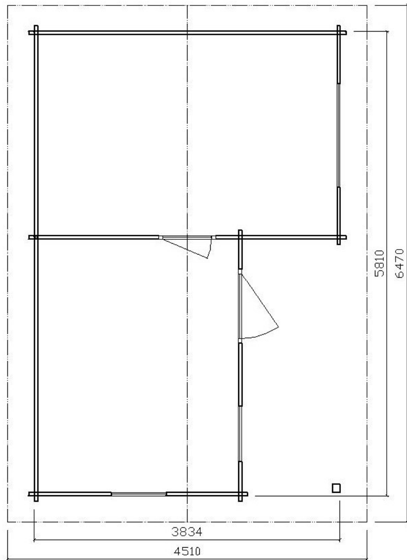
PÔDORYS
