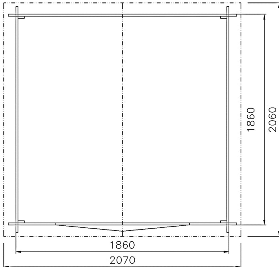
PÔDORYS
