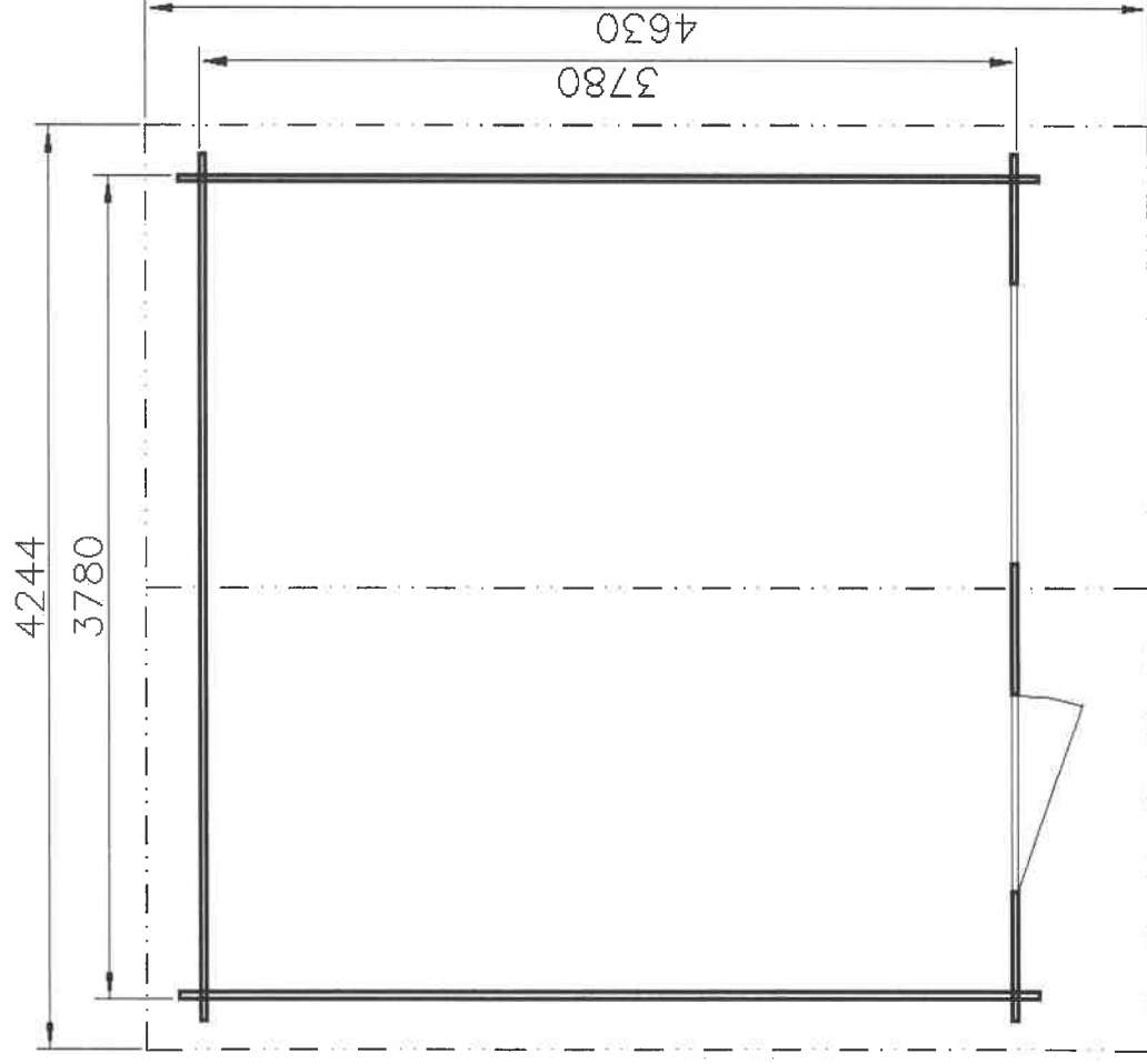
PÔDORYS
