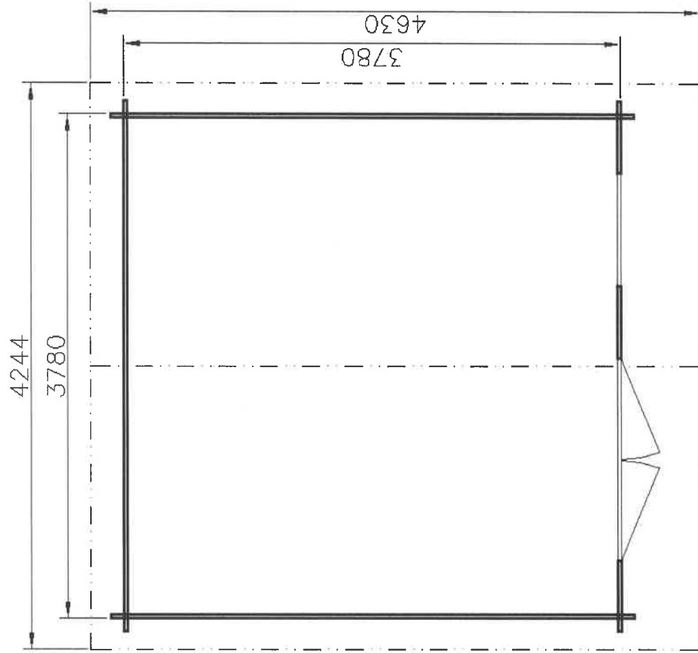
PÔDORYS
