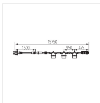
GRL 15M15E27-B
