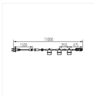
GRL 11M10E27-B
