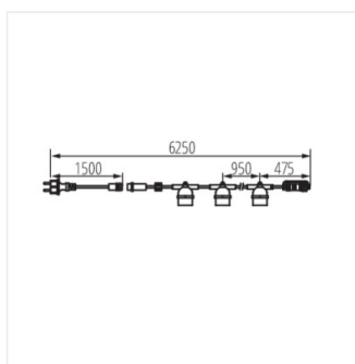
GRL 6M5E27-B
